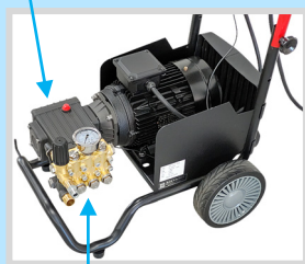
セラミックピストン 水平三連プランジャー型ポンプ
